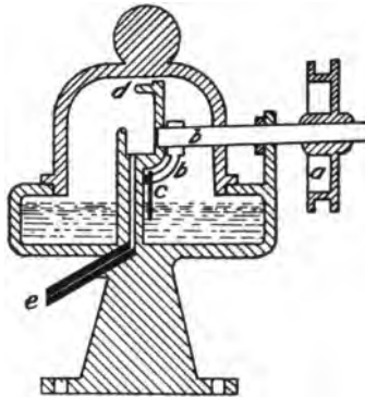
FIG. 45.—Mechanical Lubricator.
